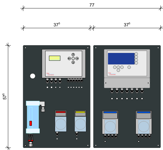
Dosieranlage DesOx 3.0, FlocDos und Steuerung DesOx Control auf System-Montage-Platte
